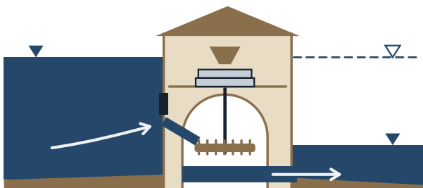
Figura 1. Dos horas tras la pleamar: el estanque mueve el rodezno y la ría ha quedado por debajo de la línea discontinua.
